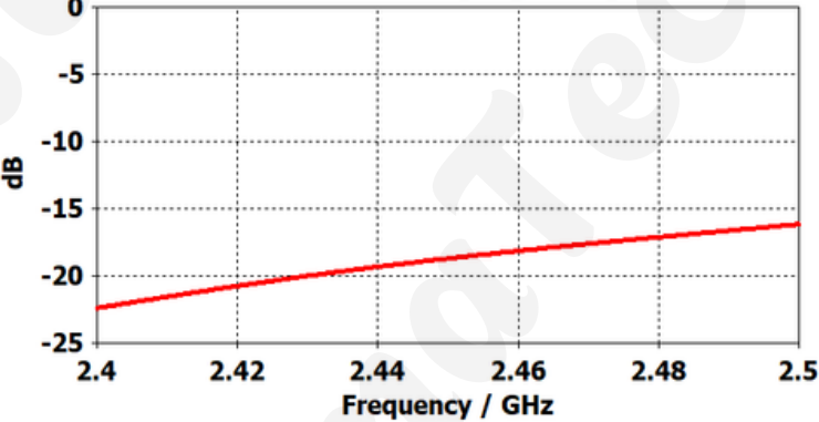
S-Parameters [Magnitude]
